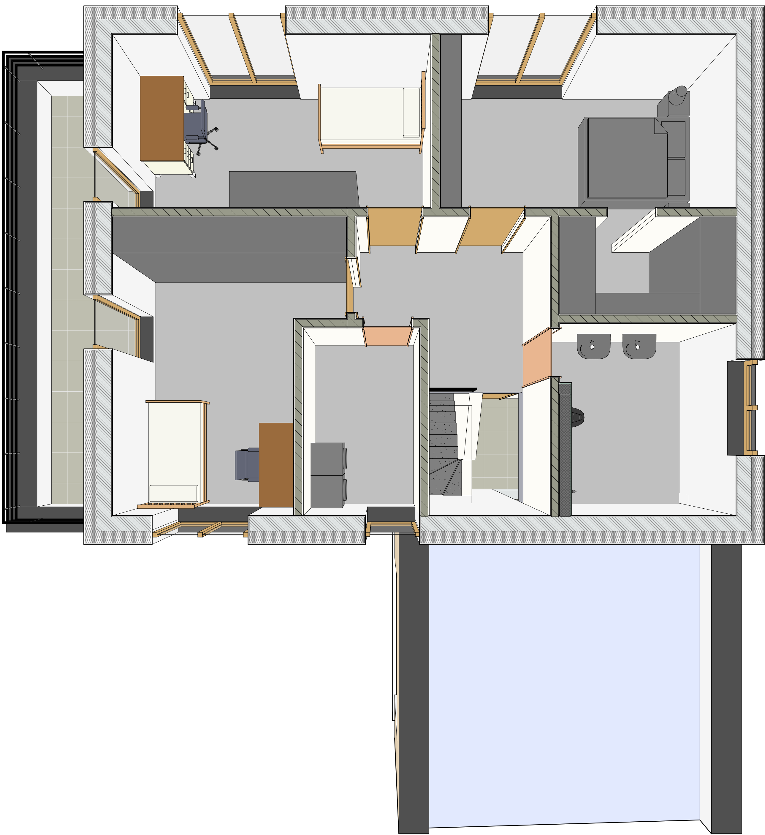
RZUT PIĘTRA
